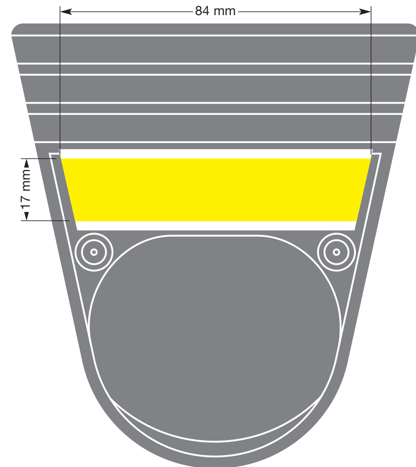
Aufsicht voorzijde front vue du haut
