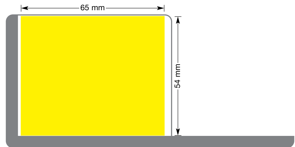
Frontansicht (linke Seite) linker voorzijde frontview (left side) vue du haut (côte gauche)
